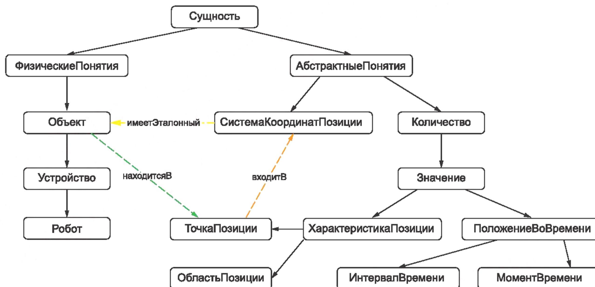
Рисунок 6 — Таксономия основных концептуальных понятий онтологии POS, соответствующих действиям робота в физической среде
