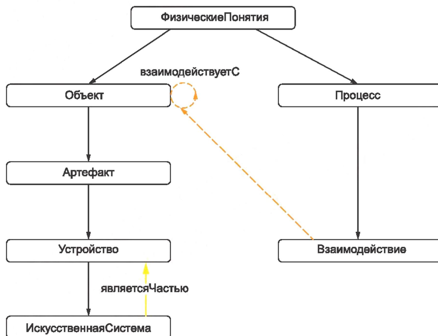
Рисунок 3 — Таксономия понятий ИскусственнаяСистема и Взаимодействие онтологии CORAX
