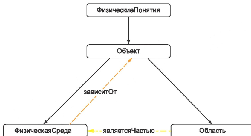
Рисунок 4 — Таксономия понятия ФизическаяСреда онтологии CORAX
