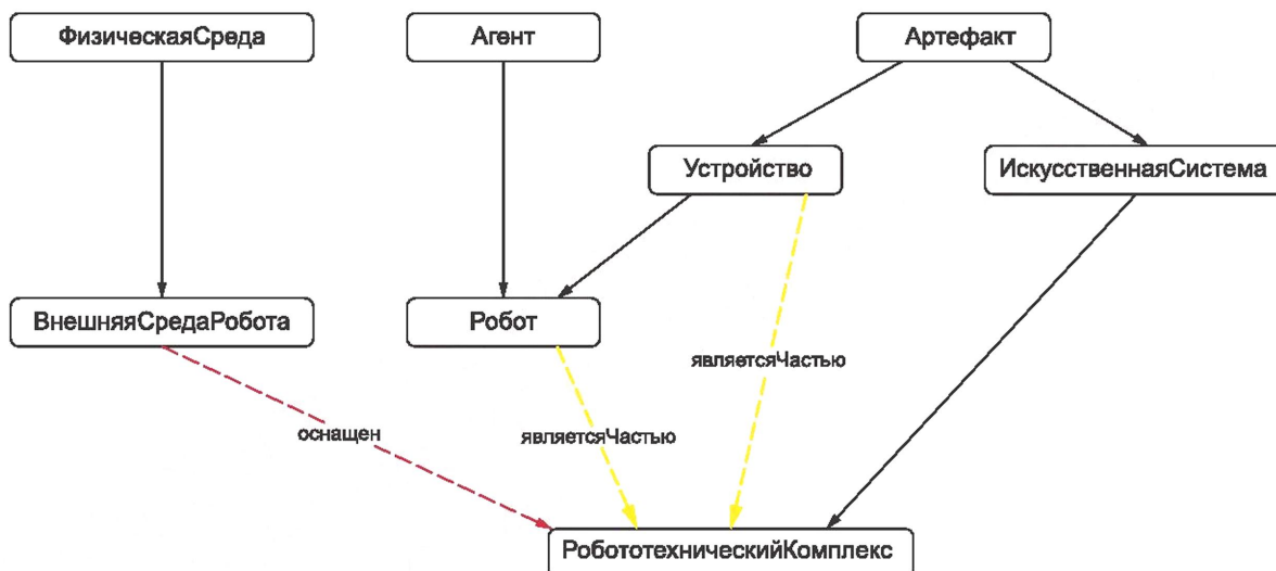
Рисунок 5 — Связь понятий ФизическаяСреда , ВнешняяСредаРобота , РобототехническийКомплекс
