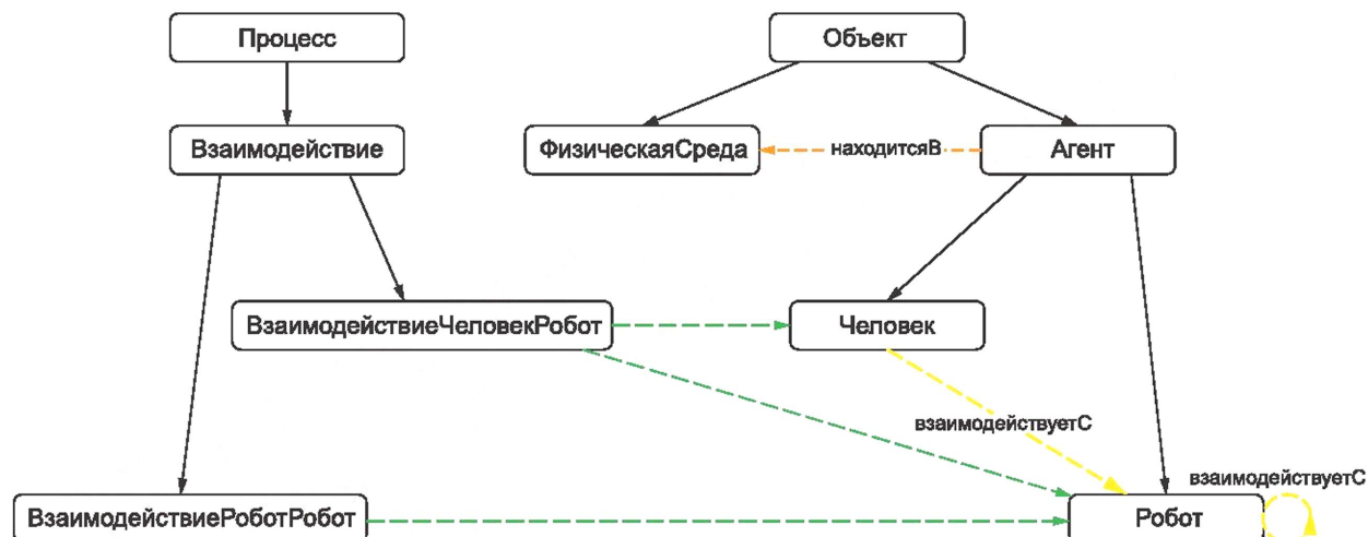
Рисунок 7 — Таксономия понятий ВзаимодействиеЧеловекРобот и ВзаимодействиеРоботРобот
