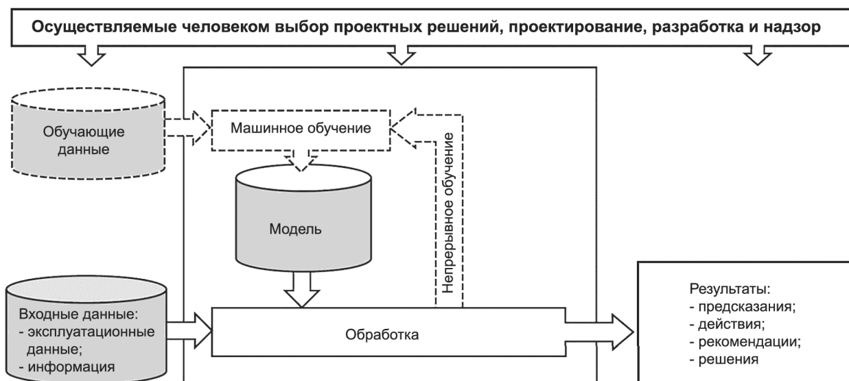
Рисунок 5 - Функциональное представление системы ИИ
