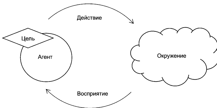
Рисунок 1 - Парадигма агента
