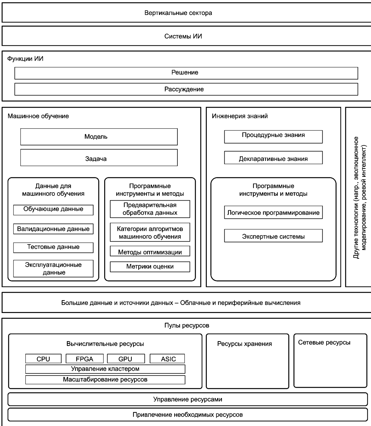
Рисунок 6 - Экосистема ИИ
