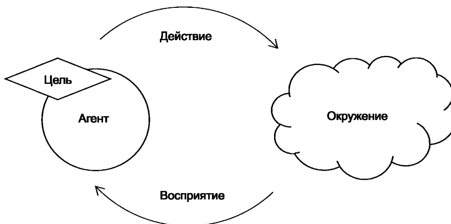
Рисунок 1 — Парадигма агента
