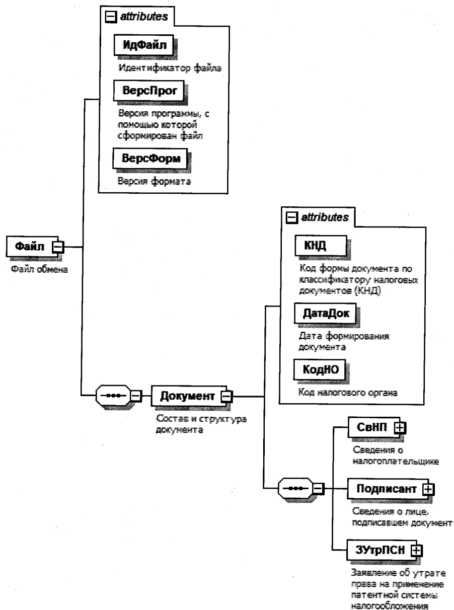
Рисунок 1. Схема структуры файла обмена
